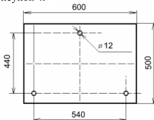
Установочные размеры.
